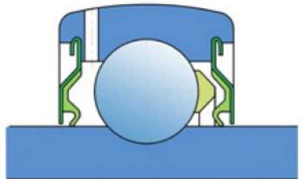
Уплотнение 2RS
