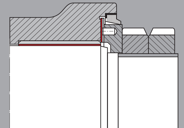
Abbildung 3.3.3 – Spezialdichtung Figure 3.3.3 – Special seal
